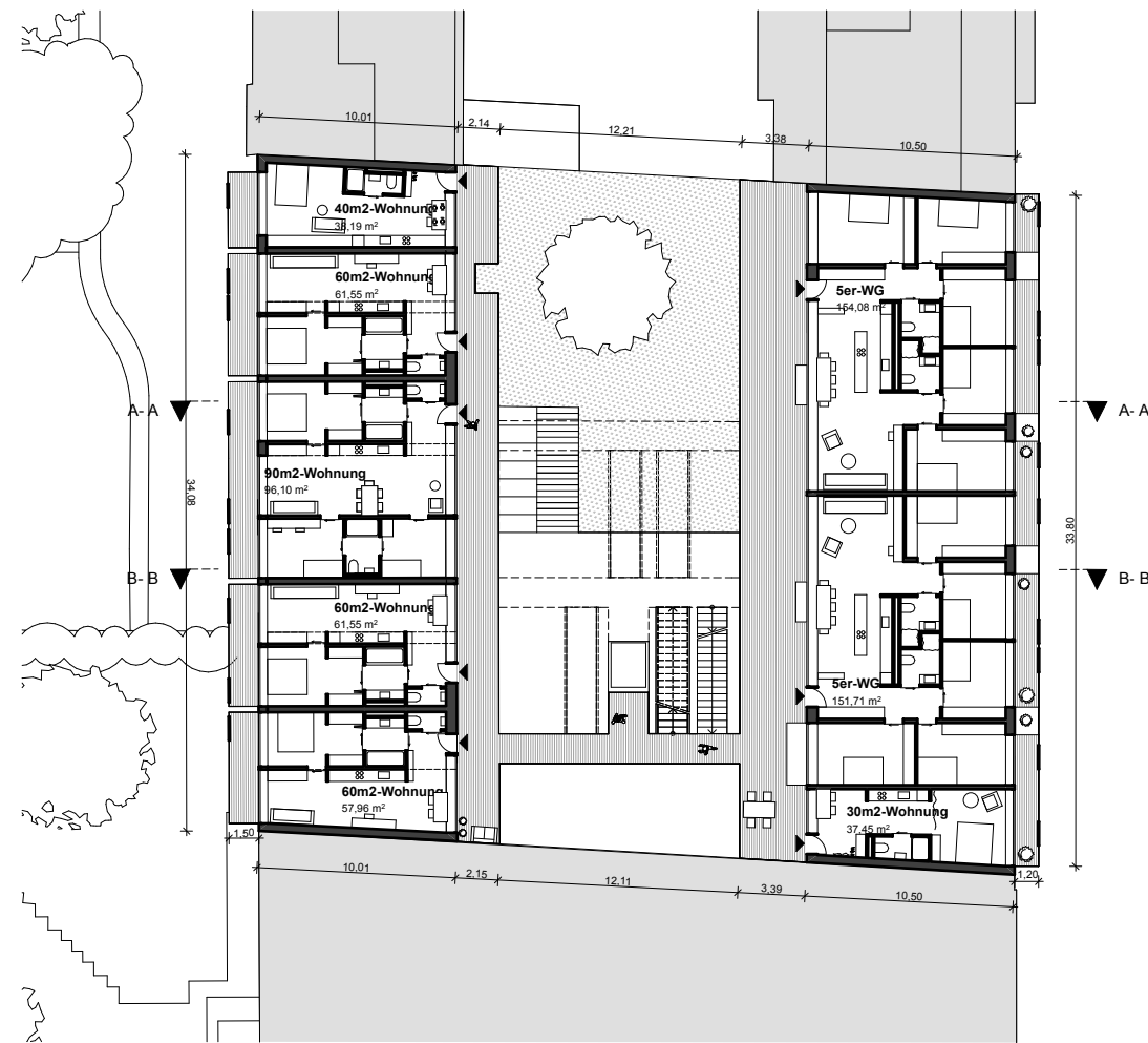
Grundriss 1.OG
