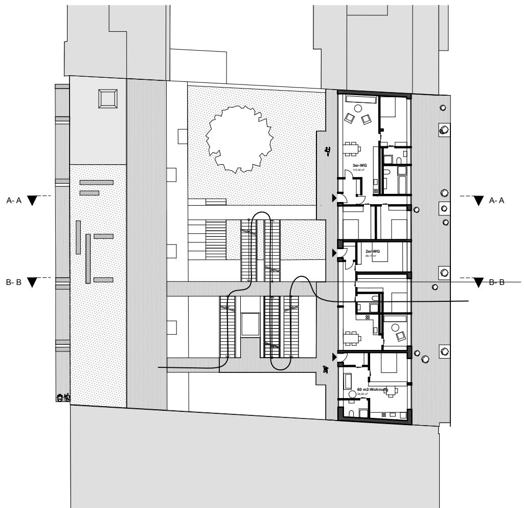
Grundriss 5. OG
