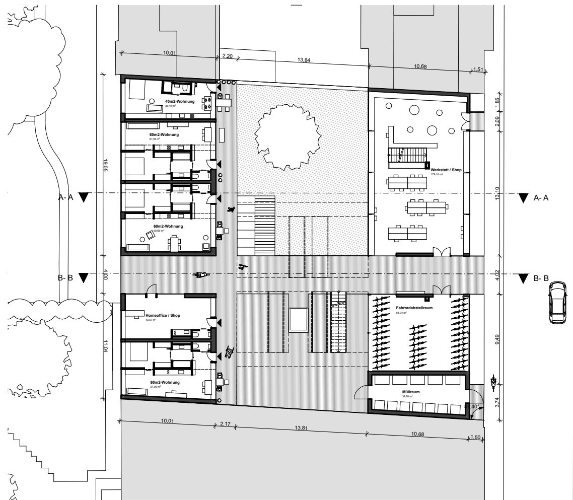
Grundriss EG
