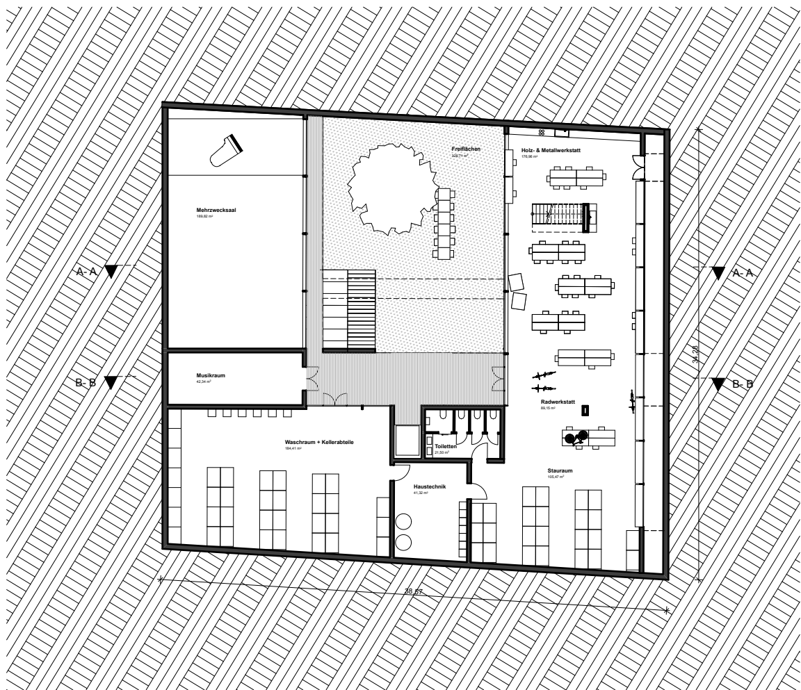
Grundriss 1.UG
